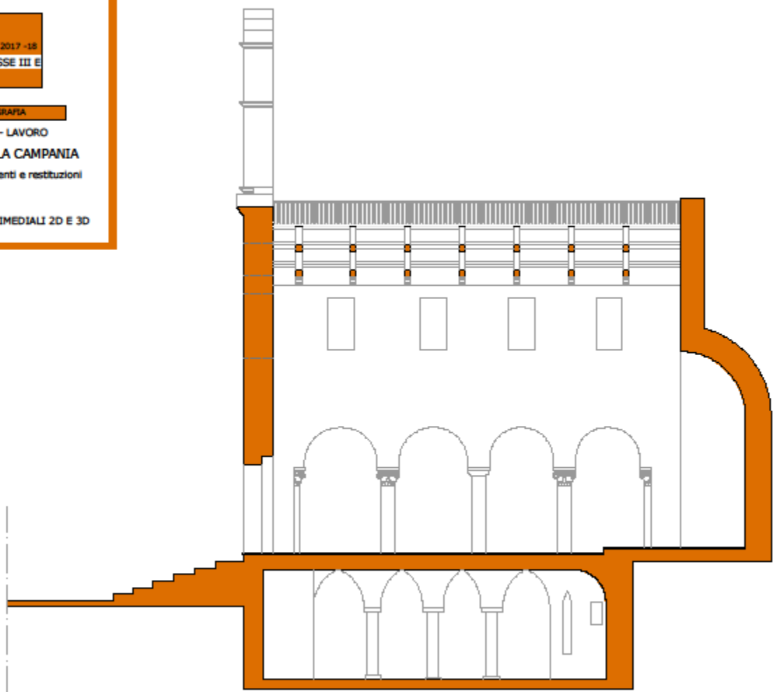
Sezione longitudinale scala 1 : 50
