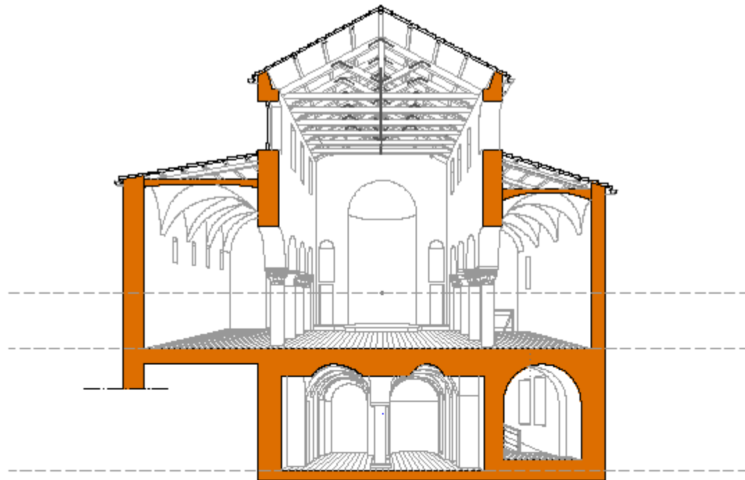
Prospettiva centrale chiesa superiore e ipogeo
